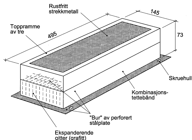
Fig. 1 Sealmaster brannhemmende lufteventil. Prinsipiell oppbygning. Brutto mål inkl. flens er 185x535x73 mm.
