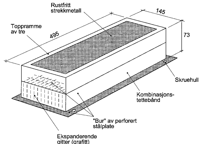
Fig. 1 Sealmaster brannhemmende lufterventil. Prinsipiell oppbygning. Brutto mål inkl. flens er 185x535x73 mm.
