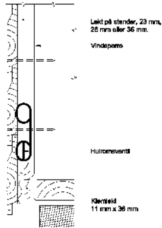
Montering i utlektet horisontal kledning - M 1:2
